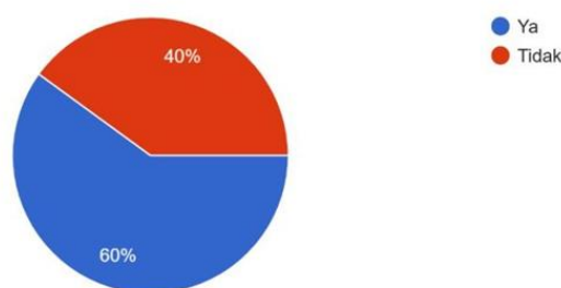
Gambar 4 . Pertanyaan kuesioner 2
