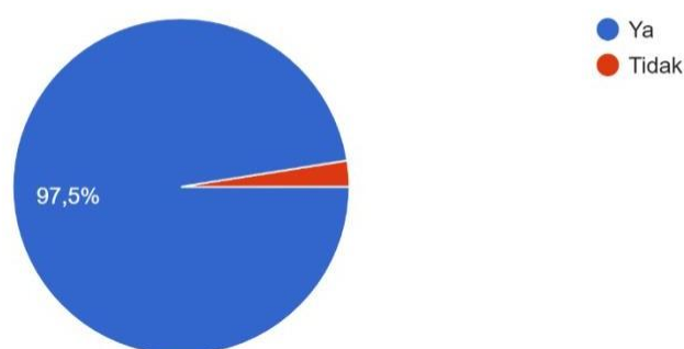
Gambar 3 . Pertanyaan Kuesioner 1
